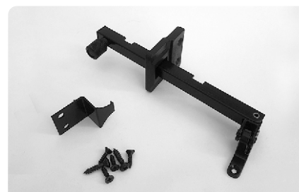
COD. 563 BRAZO DE EMPUJE FRANCA TANIT COPLANAR 20 NEGRO TANIT POR UNIDAD
