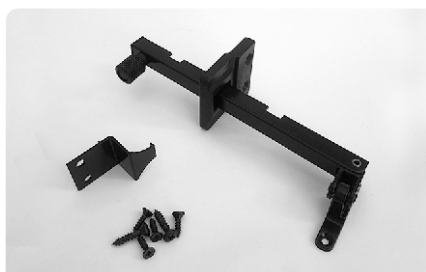
COD. 564 BRAZO DE EMPUJE FRANCA TANIT COPLANAR 30 NEGRO TANIT POR UNIDAD
