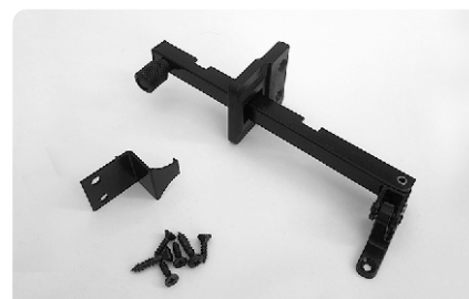
COD. 765 BRAZO DE EMPUJE AXIAL COPLANAR 40 NEGRO AX POR UNIDAD
