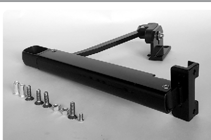
COD. 1680 BRAZO DE EMPUJE CORTO 224 MM NUMIXA NEGRO POR UNIDAD
