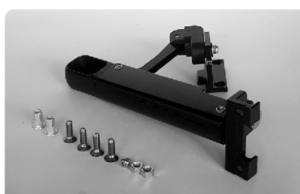
COD. 1679 BRAZO DE EMPUJE CORTO 160 MM NUMIXA NEGRO POR UNIDAD
