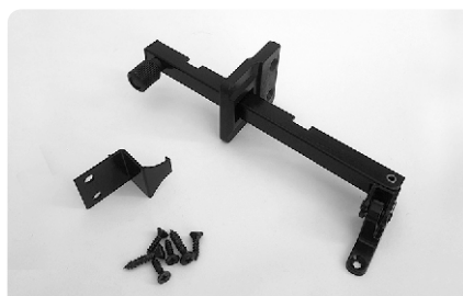
COD. 566 BRAZO DE EMPUJE AXIAL COPLANAR 30 NEGRO AX POR UNIDAD
