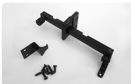
COD. 565 BRAZO DE EMPUJE FRANCA TANIT COPLANAR 40 NEGRO TANIT POR UNIDAD
